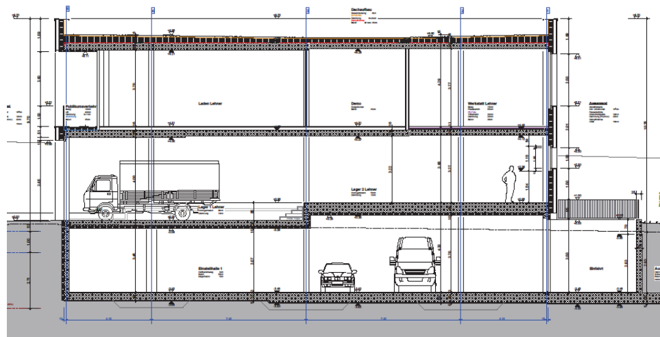
Querschnitt
